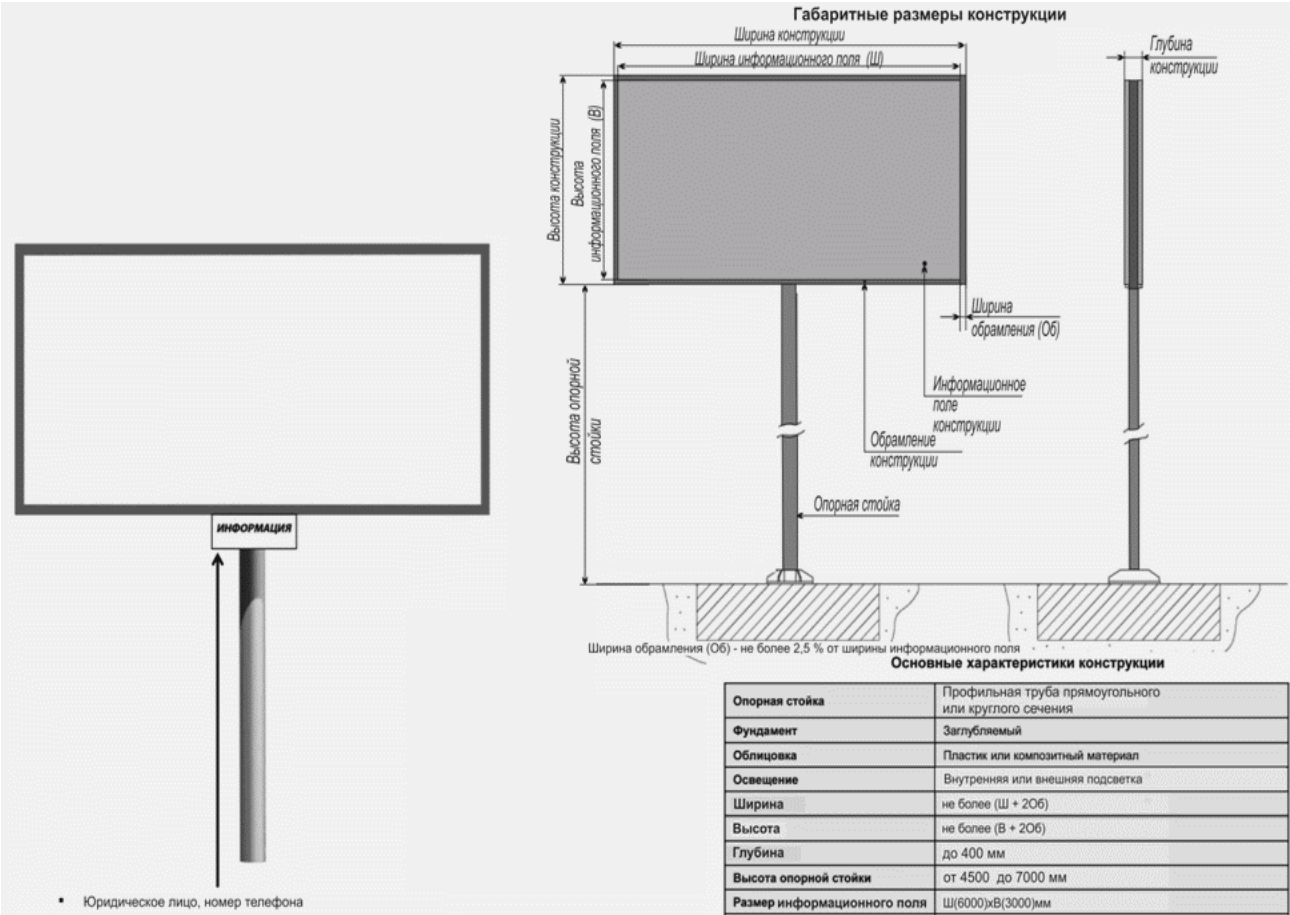
Варианты размещения опорной стойки щита 6 х 3 м
