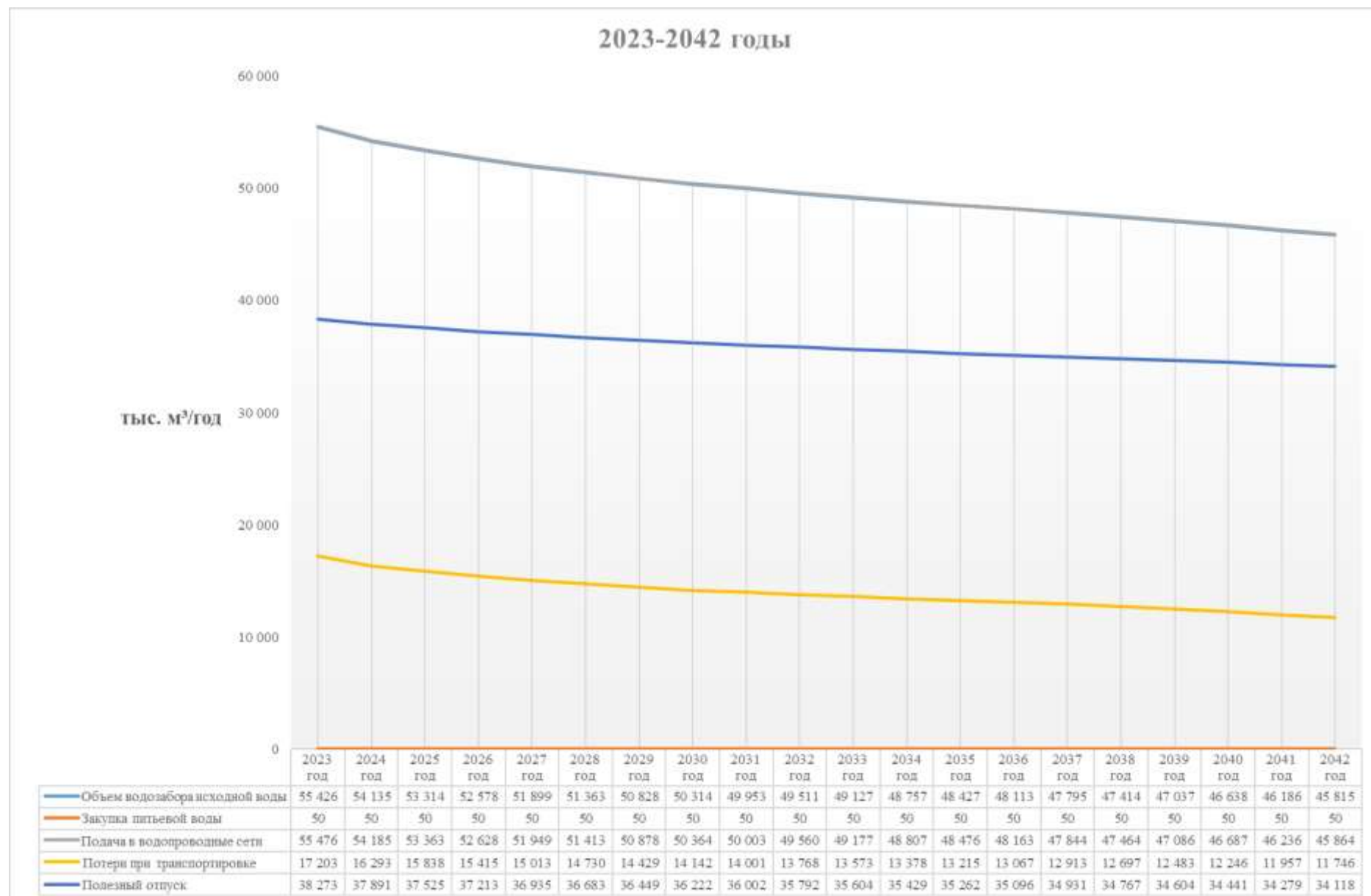
Рисунок 3.3 – Сводные прогнозные балансы водоснабжения питьевой водой ООО «РВК-Липецк» по г. Липецку на период 2023-2042
