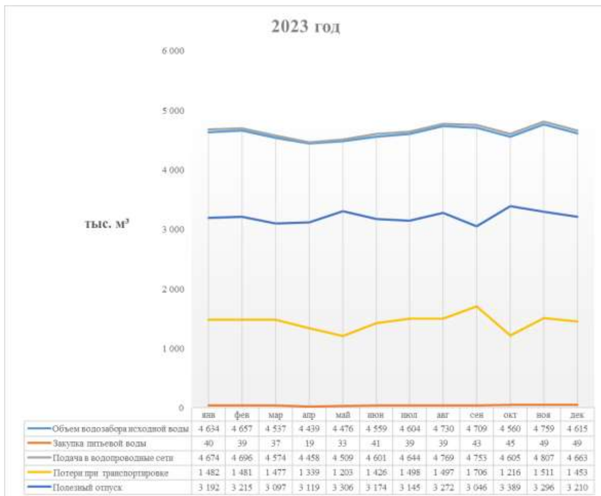
Рисунок 3.1 – Общий баланс подачи и реализации воды за 2023 год по ООО «РВК-Липецк»
