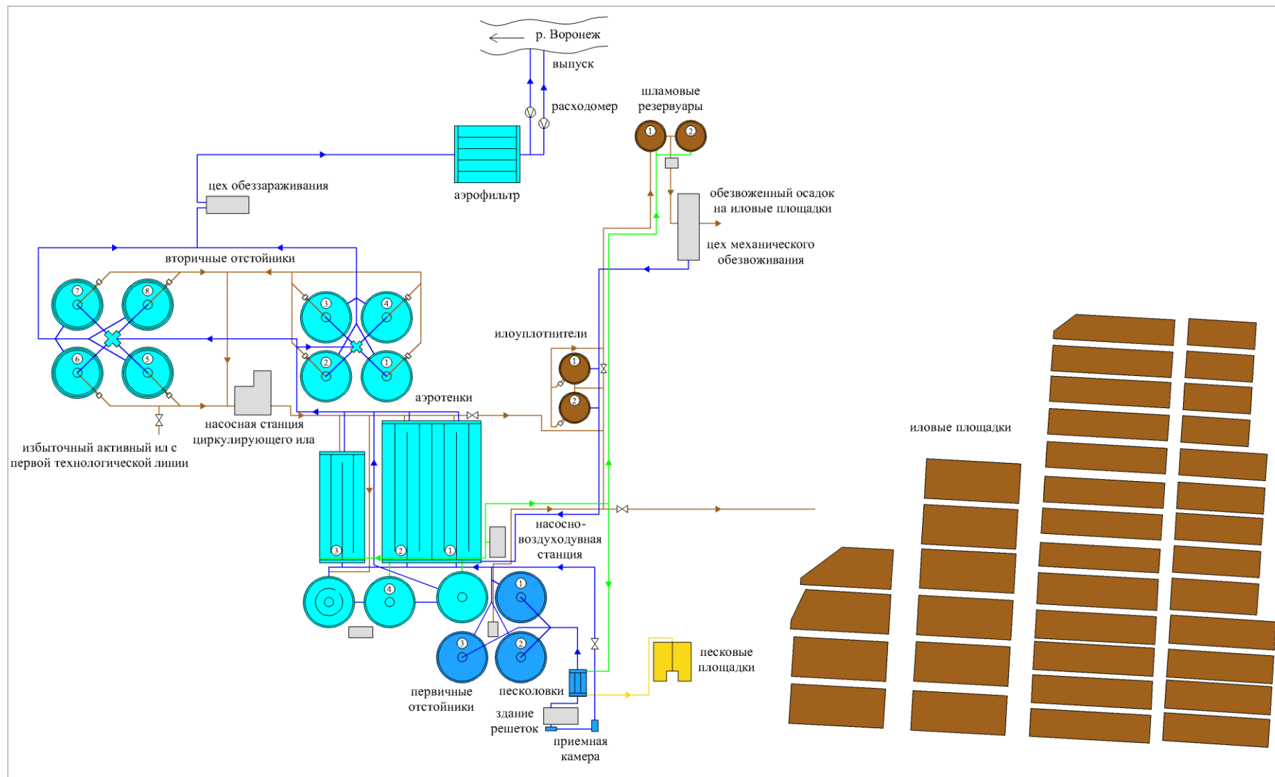
Рисунок 2-2 – Технологическая схема технологической линии очистных сооружений МУП «ЛиСА»
