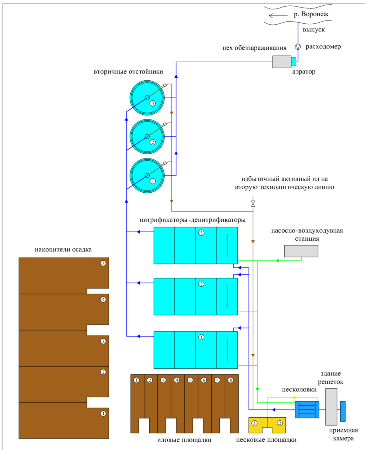
Рисунок 2-3 – Технологическая схема локальных очистных сооружений ПАО «НЛМК»
